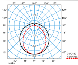
So-Tube G3 D/H2 DW 20-830 ETDD 05
