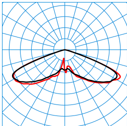
Publisca P2-RB6L-LRA/2400-730 3G1S ET (CLO end value) TX300516 ■ C0 - C180 ■ C90 - C270 DIN 5040: A20 UTE: 1,00 J DLOR: 100 % ULOR: 0 % CEN Flux Code: 20 57 98 100 100
