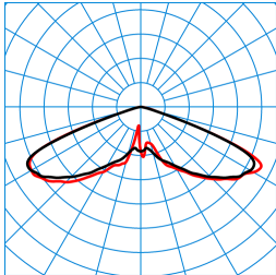
Publisca P2-RB6L-LRA/2400-730 3G1S TX047897 ■ C0 - C180 ■ C90 - C270 DIN 5040: A20 UTE: 1,00 J DLOR: 100 % ULOR: 0 % CEN Flux Code: 20 57 98 100 100
