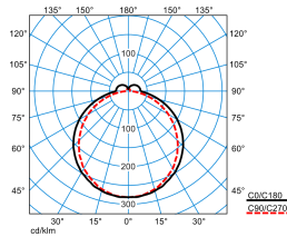
Olisq LWD2 DW 60-830 ETBLE +CAS-S IP54
