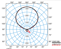
Luceos S-T PAW-IL 300-8TW ETDI 03+LLWP (DWW) (LEO1)
