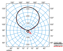
Luceos S-T PAW-IL 300-8TW ETDI 03+LLWP (DCW) (LEO1)
