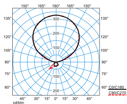
Luceos S-T PAW-IL 300-8TW ETDI 03+LLWP (DWW) (LEO2)
