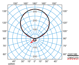
Luceos S-T PAW-IL 300-8TW ETDI 03+LLWP (DSU) (LEO2)
