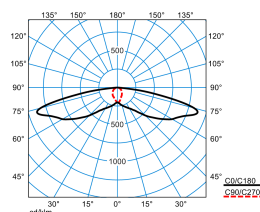
LIQ 50N-SB3L-LR/1800-722 2G1 ET (CLO end value)
