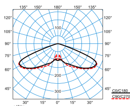
Publisca P2-RB6L-LR/4200-740 6G1S ET (CLO end value) TX301411
