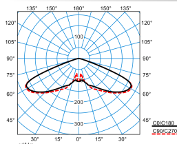
Publisca P2-RB6L-LR/4200-740 6G1S TX047873
