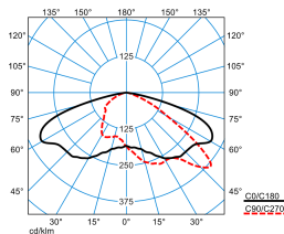
LnPlus 40-AB7L-SLR1/2200-722 2G1 ET (CLO end value)
