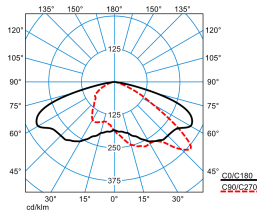
LnPlus 40-AB7L-SLR1/2200-722 2G1 ET (CLO initial value)
