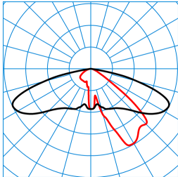
Publisca P1-AB2L-LRA/3800-740 6G1S TX047569 ■ C0 - C180 ■ C90 - C270 DIN 5040: A30 UTE: 1,00 G DLOR: 100 % ULOR: 0 % CEN Flux Code: 35 74 97 100 100
