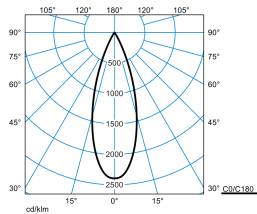
E-Line PRO 78 Lentyp L-FL 40-840 M35 ETBLE 05 05
