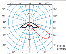
LnPlus 40-AM19L/10000-740 8G1 ETDD (CLO end value) TX377309
