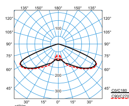
Publisca P1-RB6L-LR/5100-730 6G1S ET (CLO initial value)
