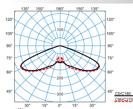
Publisca P1-RB6L-LR/5100-730 6G1S
