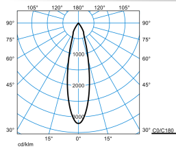
AgiraP G2 RF-MF 60-EW M50 ET 01
