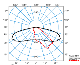
LIQ 50N-AB2L-LR/6800-722 6G1 ET (CLO end value)
