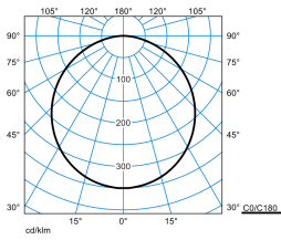
Olisq RWD1 DW 20-840 ET IP54 PC + Olisq RWD1 ZVF 01
