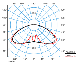
Publisca P1W-RBT-LR/1800-730 2G1S
