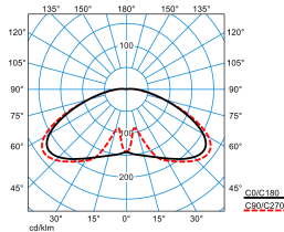
Publisca P1W-RBT-LR/1800-730 2G1S ET (CLO initial value)
