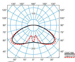
Publisca P1W-RBT-LR/1800-730 2G1S ET (CLO end value)
