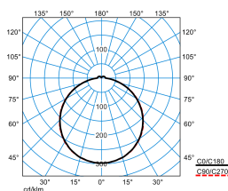
Olisq QWD2 DW 35-840 ET HFS IK + Olisq QWD2 ZDR 1/2 03
