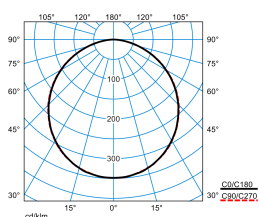
Olisq QWD2 DW 35-840 ET HFS IK + Olisq QWD2 ZDR 1/1 01 TX462044
