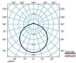
Olisq QWD2 DW 35-840 ET HFS IK TX777234
