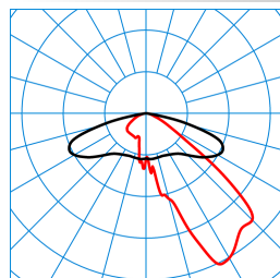
Publisca P2-AB2L/2900-730 4G1S TX047716 ■ C0 - C180 ■ C90 - C270 DIN 5040: A30 UTE: 1,00 G DLOR: 100 % ULOR: 0 % CEN Flux Code: 35 73 97 100 100
