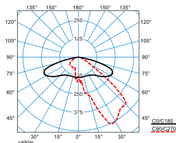
Publisca P1-AB2L-LRA/2900-730 4G1S ET (CLO end value) TX301129
