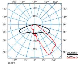
Publisca P1-AB2L-LRA/2900-730 4G1S
