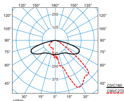
Publisca P1-AB2L-LRA/2900-730 4G1S ET (CLO end value)
