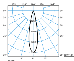
E-Line PRO 78 Lentyp L-MF 20-BC M49 ET 05 Blank
