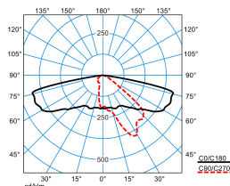
9301K AB2L-LR-SLR2/2000-740 4G3 ET (CLO end value)
