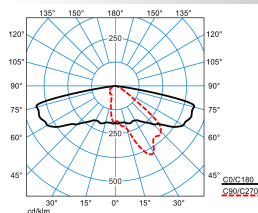
9301K AB2L-LR-SLR2/2000-740 4G3 ET (CLO initial value)
