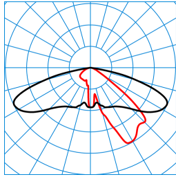
Publisca P1-AB2L/3800-730 6G1S TX047494 ■ C0 - C180 ■ C90 - C270 DIN 5040: A30 UTE: 1,00 G DLOR: 100 % ULOR: 0 % CEN Flux Code: 35 74 97 100 100
