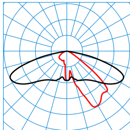
Publisca P1-AB2L/3800-730 6G1S ETDD (CLO initial value) TX301538 ■ C0 - C180 ■ C90 - C270 DIN 5040: A30 UTE: 1,00 G DLOR: 100 % ULOR: 0 % CEN Flux Code: 35 74 97 100 100
