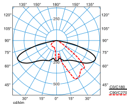
Publisca P1-AB2L/3800-730 6G1S TX047494 DIN 5040: A30 UTE: 1,00 G DLOR: 100 % ULOR: 0 % CEN Flux Code: 35 74 97 100 100
