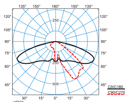
Publisca P1-AB2L/3800-730 6G1S ETDD (CLO end value) TX300924 DIN 5040: A30 UTE: 1,00 G DLOR: 100 % ULOR: 0 % CEN Flux Code: 35 74 97 100 100
