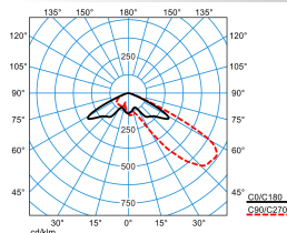
LnPlus 70-AM19L-SLR2/62000-740 48G1 ET (CLO end value) TX377733
