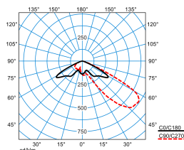
LnPlus 70-AM19L-SLR2/62000-740 48G1 ET (CLO initial value) TX377208
