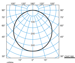
Olisq RWD4 DW 40-8TW ETBLE +CAS IP54 + Olisq RWD4 ZDR 1/1 05 (DWW)
