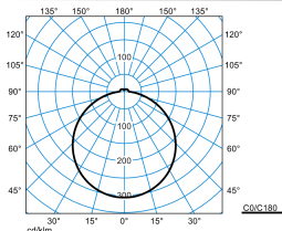
Olisq RWD4 DW 40-8TW ETBLE +CAS IP54 (DWW)
