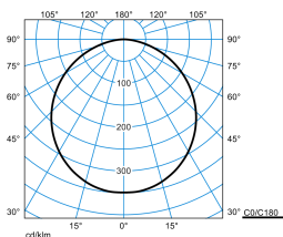
Olisq RWD4 DW 40-8TW ETBLE +CAS IP54 + Olisq RWD4 ZDR 1/1 03 (DWW)
