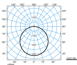
Olisq RWD4 DW 40-8TW ETBLE +CAS IP54 + Olisq RWD4 ZDR 1/2 03 (DCW)
