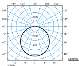
Olisq RWD4 DW 40-8TW ETBLE +CAS IP54 + Olisq RWD4 ZDR 1/2 05 (DCW)
