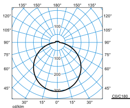
Olisq RWD4 DW 40-8TW ETBLE +CAS IP54 (DCW)
