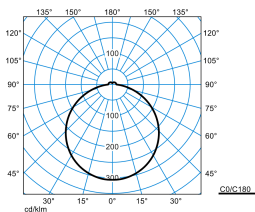
Olisq RWD4 DW 40-8TW ETBLE +CAS IP54 (DSU)
