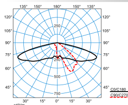
Publisca P1W-AB2L-LR/2600-740 3G1S ET (CLO initial value)
