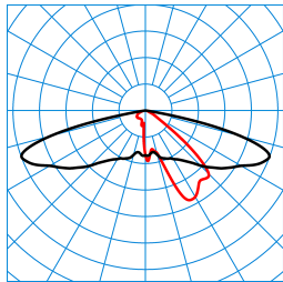
Publisca P1W-AB2L-LR/2600-740 3G1S ET (CLO end value) TX031766 ■ C0 - C180 ■ C90 - C270 DIN 5040: A30 UTE: 1,00 l DLOR: 100 % ULOR: 0 % CEN Flux Code: 32 69 96 100 100 0 33 67 0
