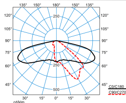
Cuvia 40-AB2L-LR/3200-740 4G1S ET
