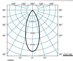
Toko RF-FL 40-BC M51 ETDD 05
