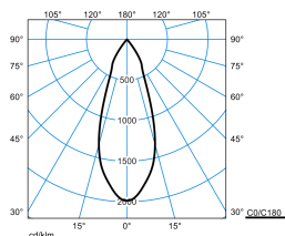
E-Line PRO 78 BV G2 RF-FL 40-EC M39 ET 05 Blank
