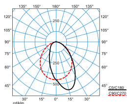
SFlow C2-L MLA LED4600-830 ETDD 01
