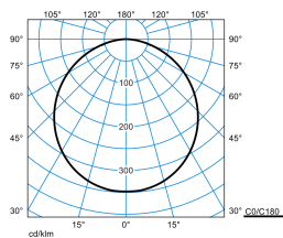
Olisq RWD2 DW 20-840 ET EB3 + Olisq RWD2 ZDR 1/1 05
