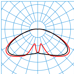
Publisca P1W-RBT-LRA/1800-740 2G1S ET (CLO end value) TX301380 ■ C0 - C180 ■ C90 - C270 DIN 5040: A20 UTE: 0.97 l + 0.03 T DLOR: 97 % ULOR: 3 % CEN Flux Code: 26 63 91 97 100 4 16 28 3
