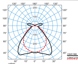
Tugra 15 PW 60-840 ETDD EB3 23 TX777230
