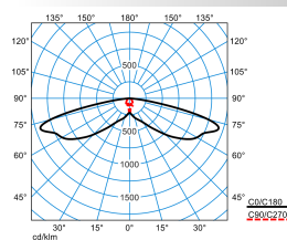
Publisca P1-SB3L/800-730 2G1S
