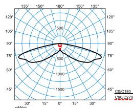
Publisca P1-SB3L/800-730 2G1S ETDD (CLO end value)
