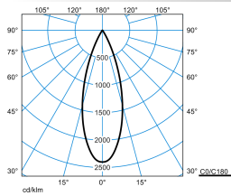
E-Line PRO 78 Lentyp L-FL 40-EW M48 ETDD 01 TX715032
