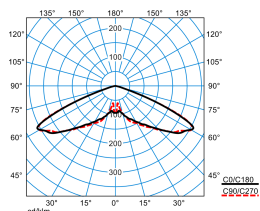
Publisca P1W-RB6L-LR/4600-740 6G1S ET (CLO end value)
