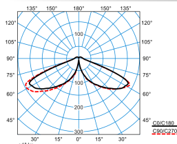
8841LS-UE 260-RB6L/2900-740 3G2 ET (CLO initial value)
