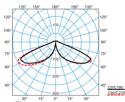
8841LS-UE 260-RB6L/2900-740 3G2 ET (CLO end value)
