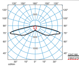
Jovie 50-SB3L-6-68-730-CLO-B
