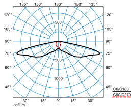
Jovie 50-SB3L-6-68-730-CLO-E
