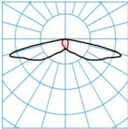
Jovie 50-SB3L-6-68-730-CLO-B
