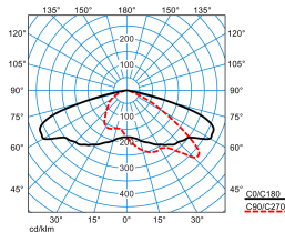
9311 AB7L-LR-SLR3/3500-740 4G3 ET (CLO end value)
