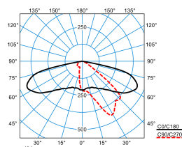
Publisca P3-AB2L-LRA/3200-740 4G1 ET (CLO end value)
