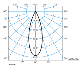
E-Line PRO 78 Lentyp L-FL 30-BF M54 ET 03 Blank
