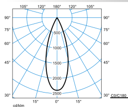
E-Line PRO 78 Lentyp L-FL 40-827 M32 ET 05 Blank
