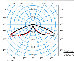
LTX L-RB6L-LRA/2600-740 3G1 ETDD
