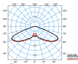
Publisca P2-RB6L-LRA/5600-740 6G1S ET (CLO initial value)
