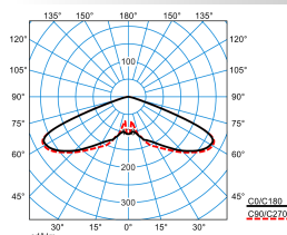
Publisca P2-RB6L-LRA/5600-740 6G1S
