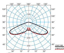
Publisca P2-RB6L-LRA/5600-740 6G1S ET (CLO end value)
