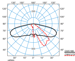
Publisca P2-AB2L-LR/2000-740 3G1S ET (CLO initial value)
