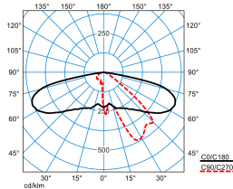
Publisca P2-AB2L-LR/2000-740 3G1S
