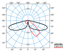
8841LS-UE 260-AB2L/2900-730 3G2 ET (CLO end value)
