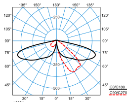
8841LS-UE 260-AB2L/2900-730 3G2 ET (CLO initial value)
