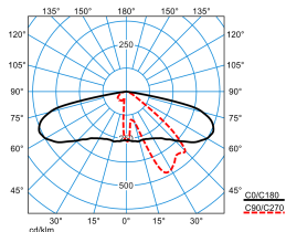
Publisca P2-AB2L-LR/1350-740 2G1S ET (CLO initial value)
