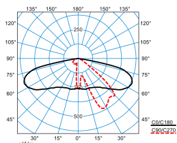
Publisca P2-AB2L-LR/1350-740 2G1S ET (CLO end value)
