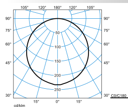
Varisto1500 15000-840 S09 ET 05 (LEO3)
