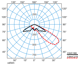
LnPlus 40-AM19L-LR/3200-730 4G1 ET (CLO end value) TX377482
