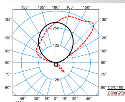
Luceos S G3 PAW-IA 170-8TW ETDS KL 05 (DWW)
