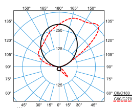
Luceos S G3 PAW-IA 170-8TW ETDS KL 05 (DSU)
