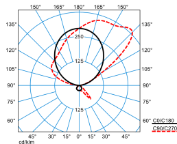
Luceos S G3 PAW-IA 170-8TW ETDS KL 05 (DCW)
