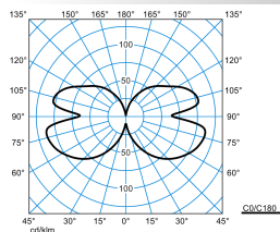
PolaroniQ W2 LED2000-830 ETDD
