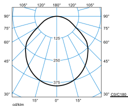
Inplana C07 OTA22 1000-840 ET 01 + C07 ZPF - T TX372707
