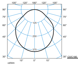
Inplana C07 OTA22 1000-840 ET 01 TX72408
