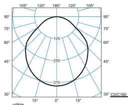
Inplana C07 OTA22 1000-840 ET 01 + C07 ZPF - T WR TX372708
